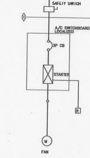
FOR FAN
